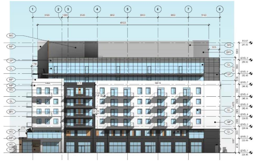
1 SOUTH ELEVATION SCALE: 1:200
