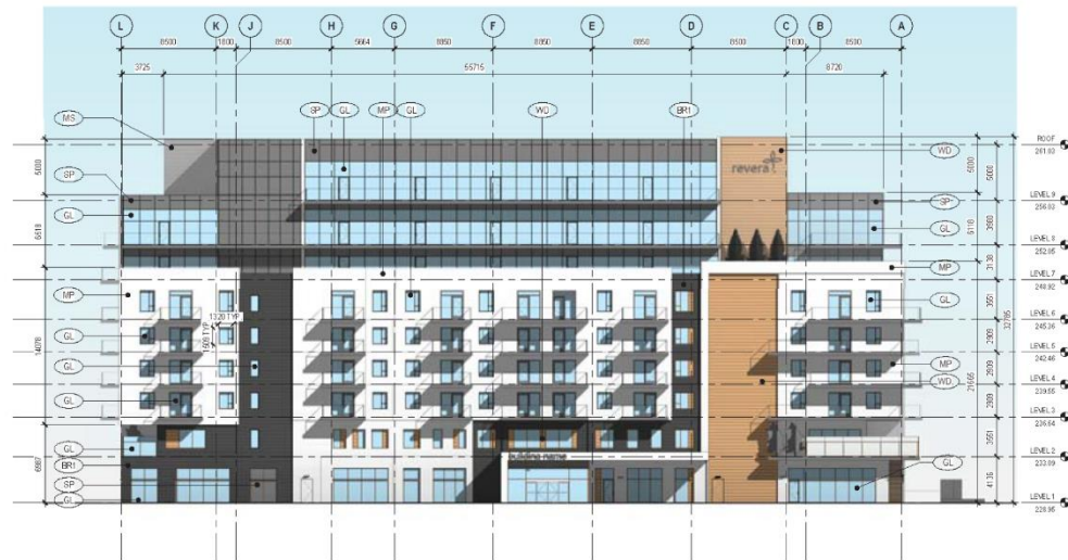
2 WEST ELEVATION SCALE: 1/200
