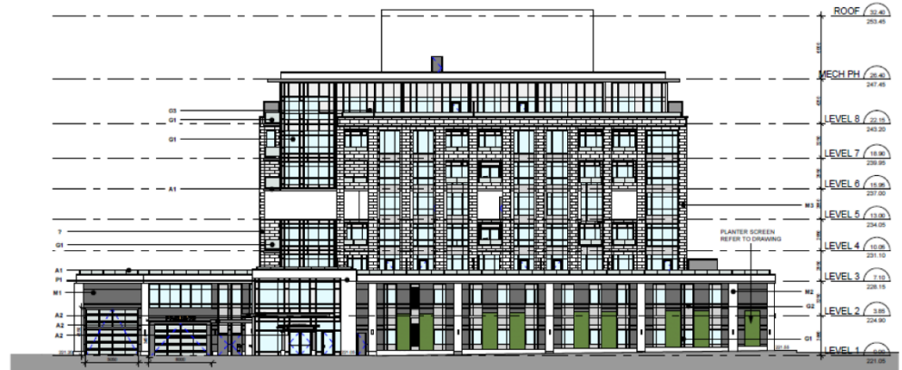
South Elevation 2 Scale: 1 : 200 A3.1
