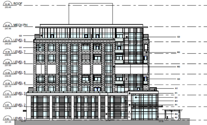
West Elevation 1 Scale: 1 : 200 A3.1
