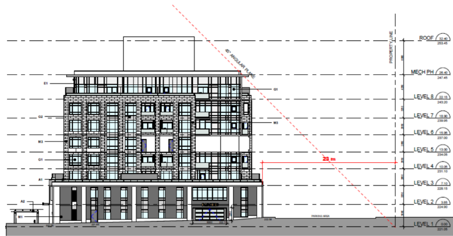
South Elevation 2 Scale: 1 : 200 A3.1
