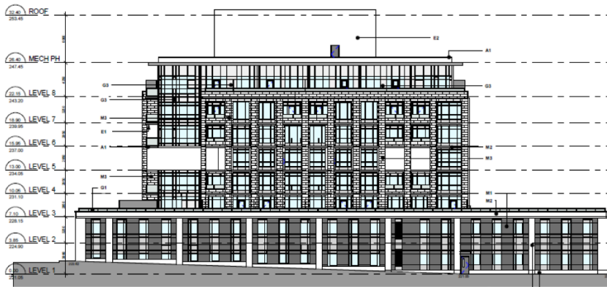
West Elevation 1 Scale: 1 : 200 A3.1
