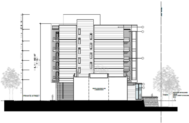
4 SOUTH ELEVATION Scale: 1:200
