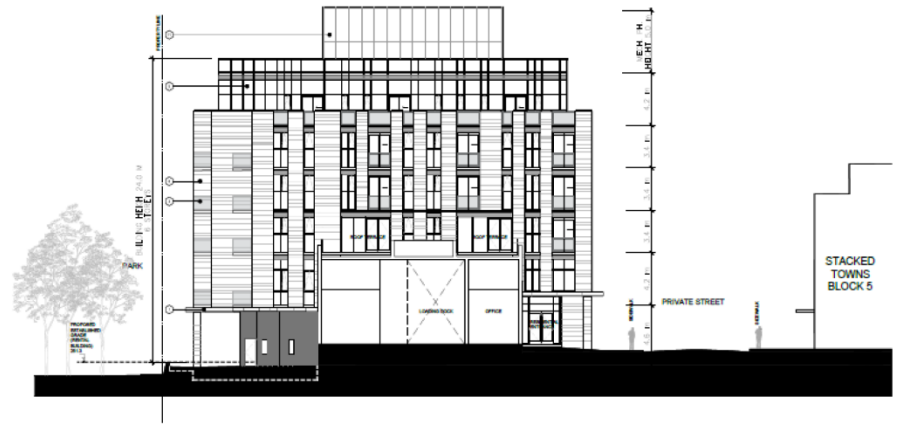
1 NORTH ELEVATION Scale: 1:200
